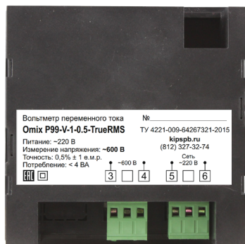
Рис. 8 – Задняя панель прибора P99
